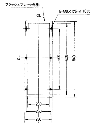
穴明寸法
