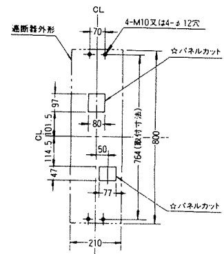
穴明寸法
