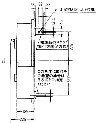
裏面形(SD)
