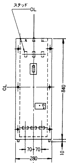
埋込形(FP)
