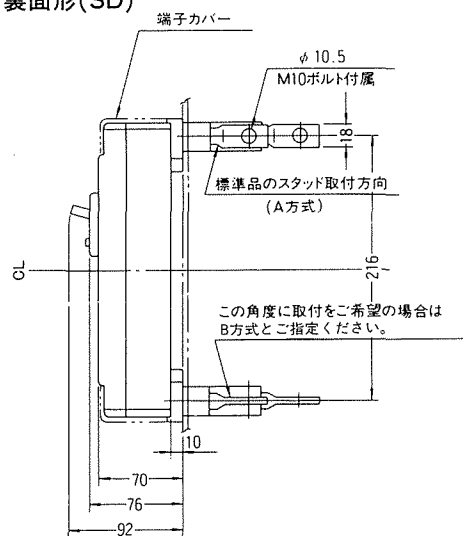
裏面形(SD)
