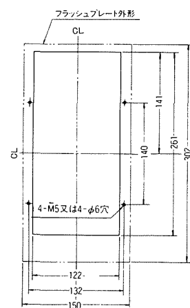
穴明寸法
