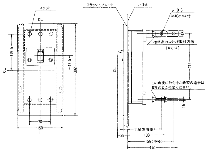
埋込形(FP)
