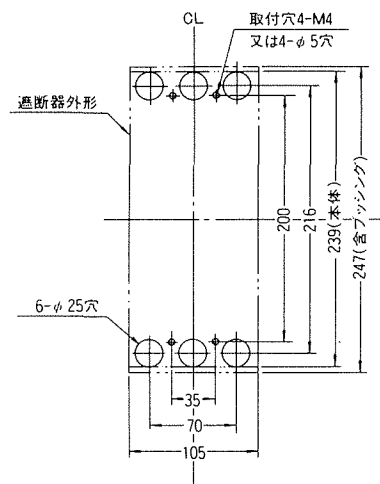
穴明寸法
