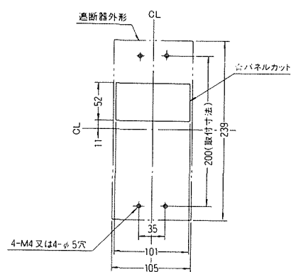
穴明寸法
