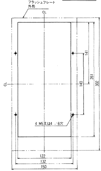
穴明寸法
