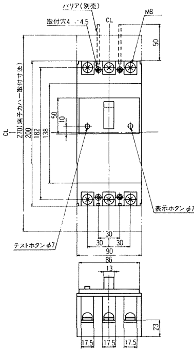
裏面形(SD)
