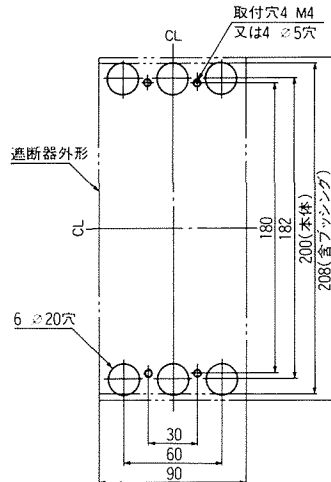
穴明寸法
