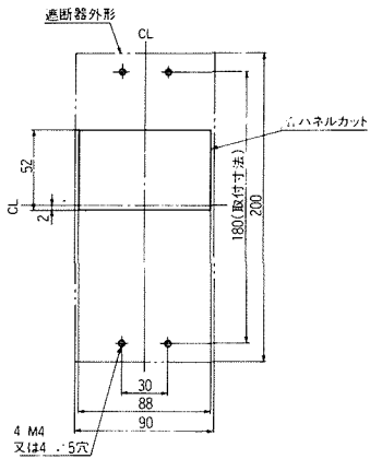
穴明寸法
