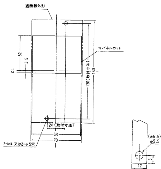
導帯加工図 (最大)
