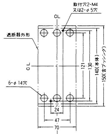
穴明寸法
