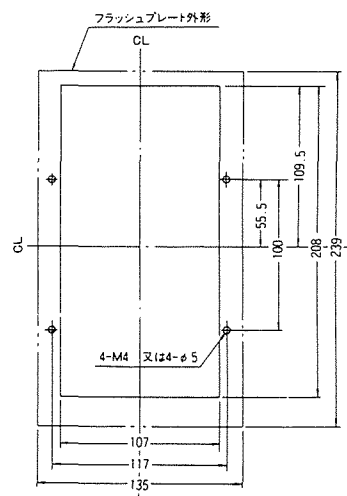
穴明寸法
