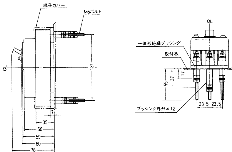
裏面形(SD)
