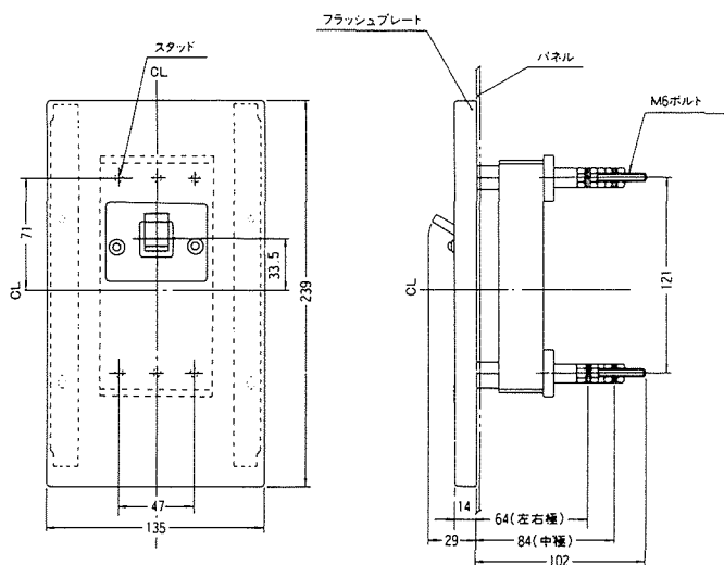
埋込形(FP)
