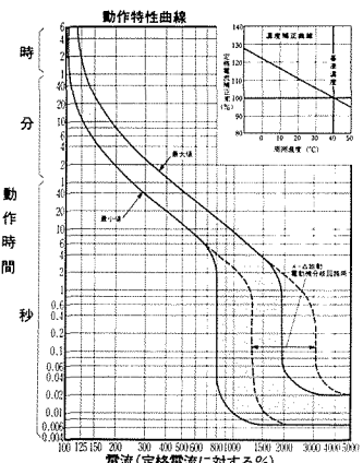
12 GB-222E・223E, GBU-223・1E
