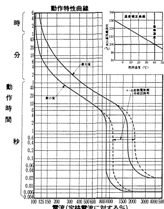
11 GB-152E・153E, GBU-153・1E
