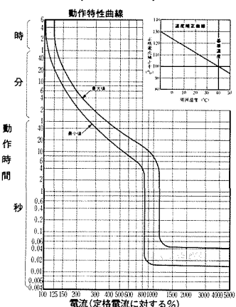
7 GB-62E・63E, GB-63・1E, GBU-63・1E
