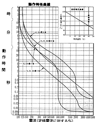
6 GB-52E・53E, GB-53・1E, GBU-53・1E
