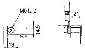
導帯, 圧着端子接続
