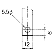
導帯加工図
