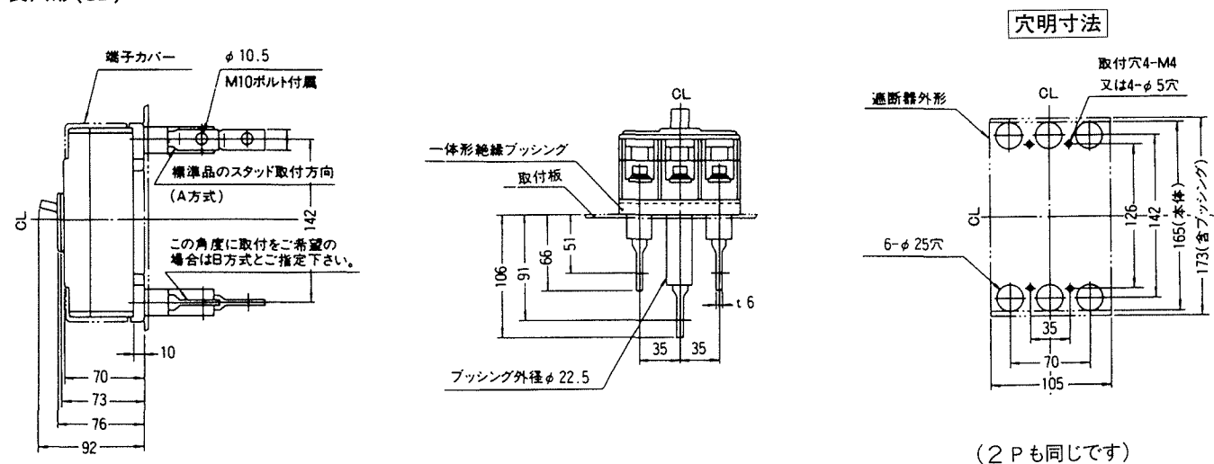
裏面形(SD)
