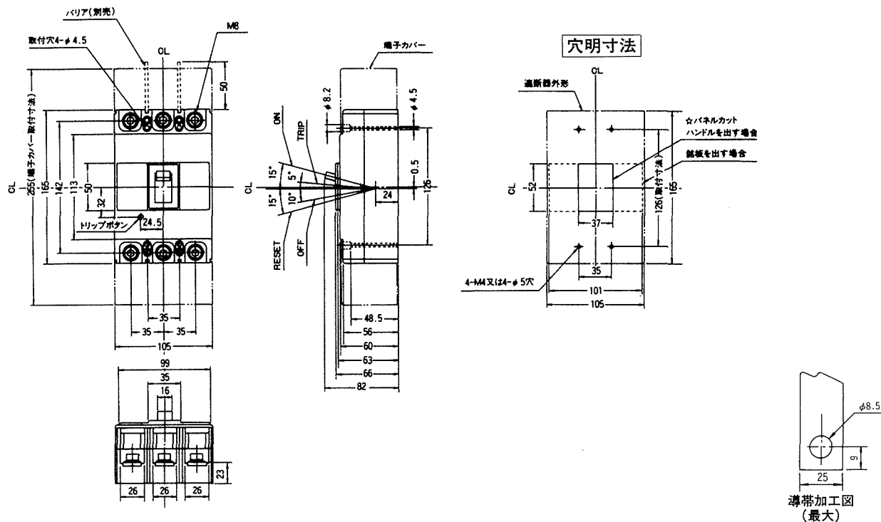
裏面形(SD)
