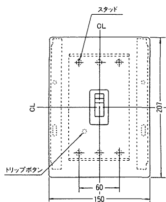
埋込形(FP)
