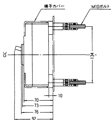
裏面形(SD)
