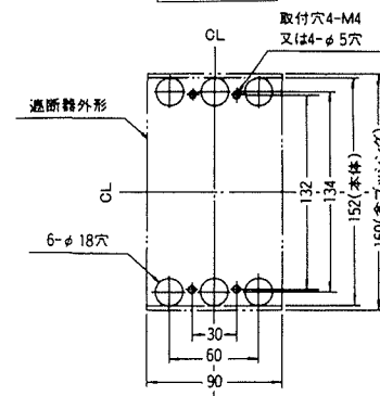
穴明寸法
