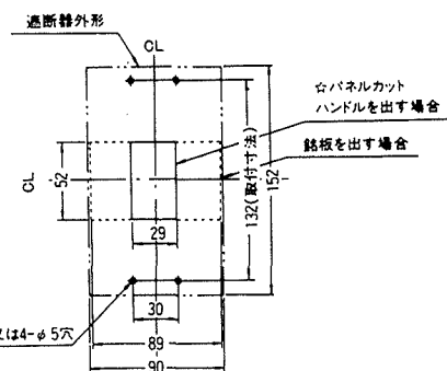
穴明寸法
