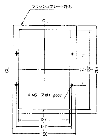
穴明寸法
