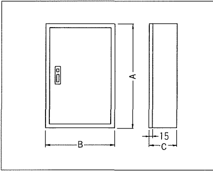
■外形寸法図(屋内用)
