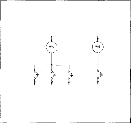
■回路図(B)
