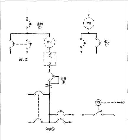
■回路図(A)
