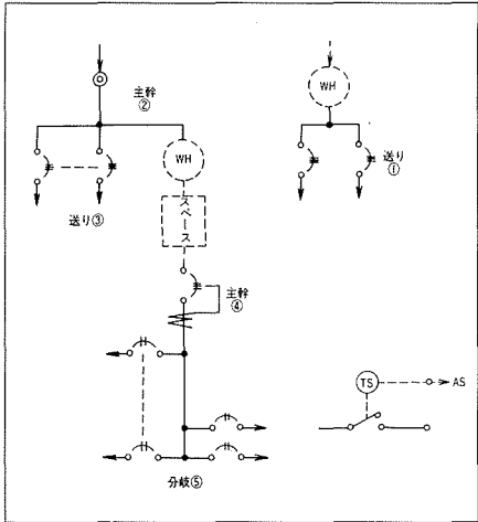
■回路図(B)
