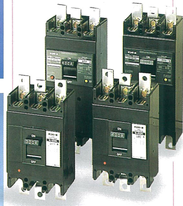
●配線用遮断器 ●漏電遮断器
