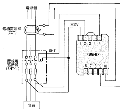
A) 制御電源を回路から取る場合
