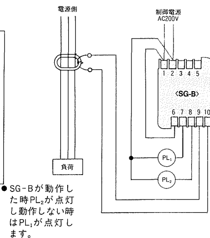
C) 警報装置を取付ける場合
