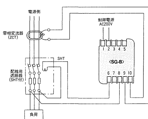
B) 制御電源を別から取る場合
