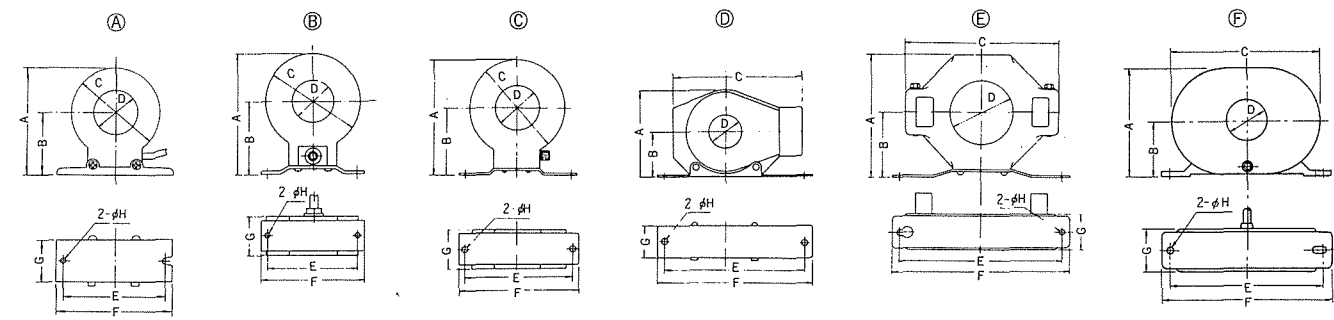
外形寸法図
