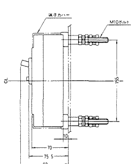
裏面形
