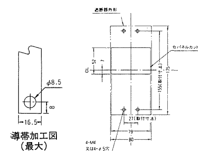
穴明寸法
