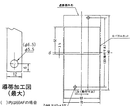
穴明寸法
