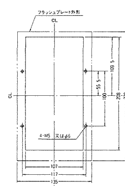
穴明寸法
