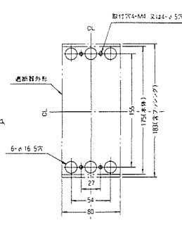
穴明寸法
