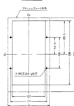
穴明寸法
