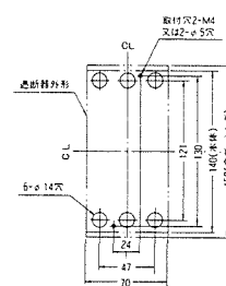
穴明寸法
