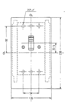
埋込形
