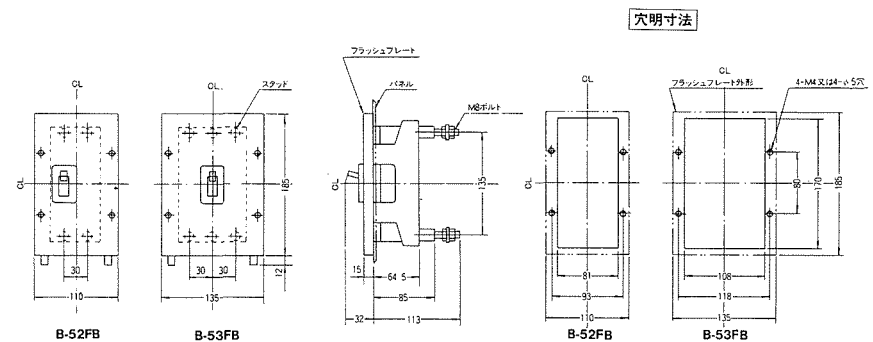
埋込形
