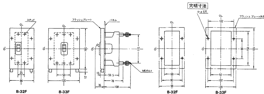
埋込形
