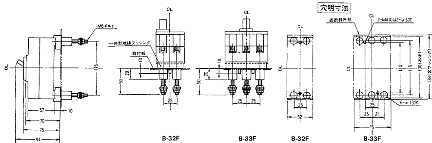
裏面形
