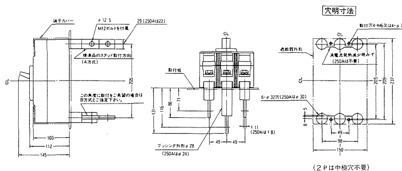
裏面形
