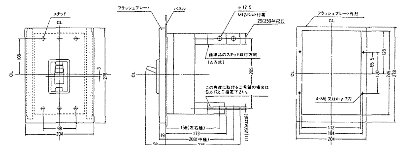
埋込形
