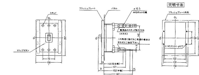
埋込形
