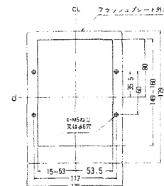
穴明寸法
