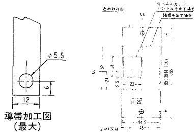
穴明寸法
