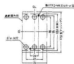
穴明寸法
