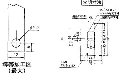
穴明寸法
