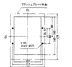
穴明寸法
