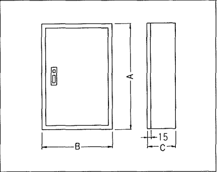
■ボックス構造 単位：mm
