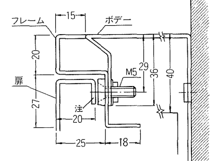
■ボックス構造 単位：mm
