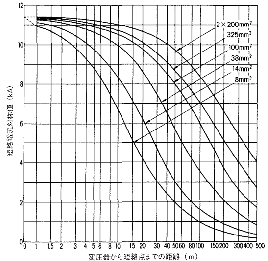
付図15 三相変圧器容量500kVA, 二次電圧415V
