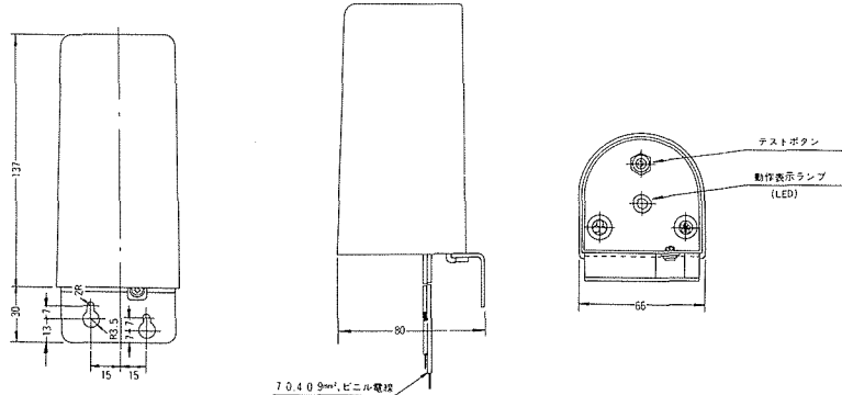
■S-2型, SOR-2型外形寸法図
