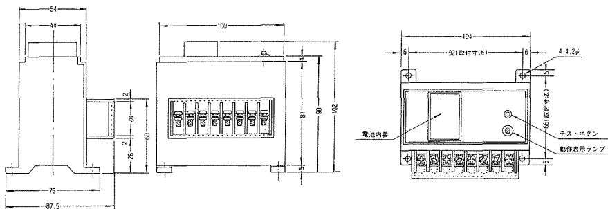
■S-2型, SOR-2型外形寸法図
