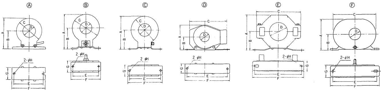
■変流器外形寸法表
