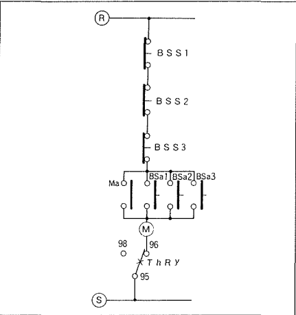
1. 操作回路図
