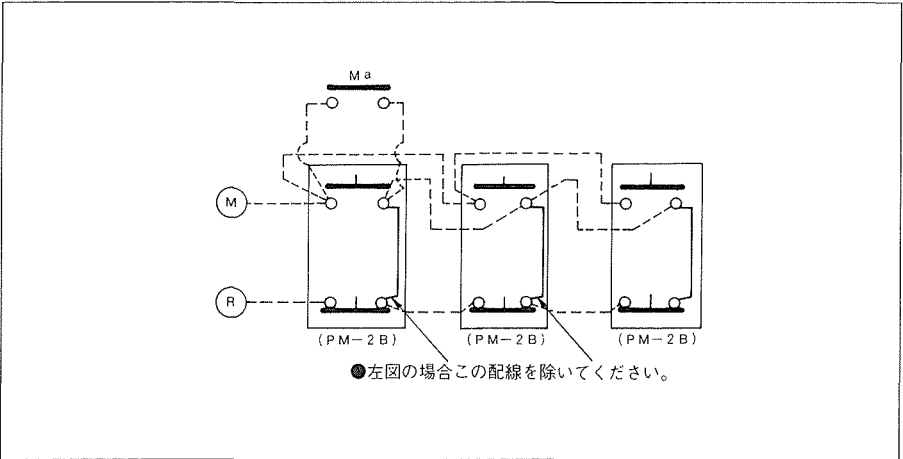
2. 結線図
