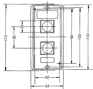
■外形寸法図
