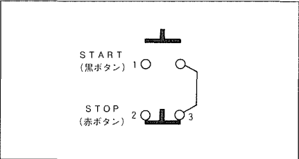
■接点構成図
