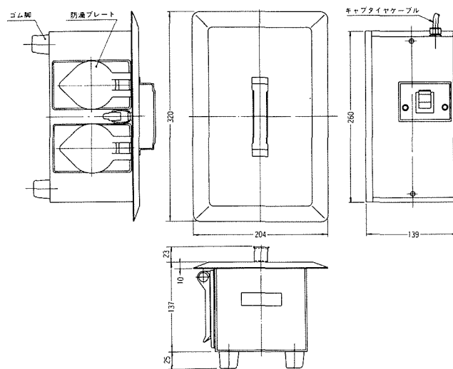
■外形寸法図
