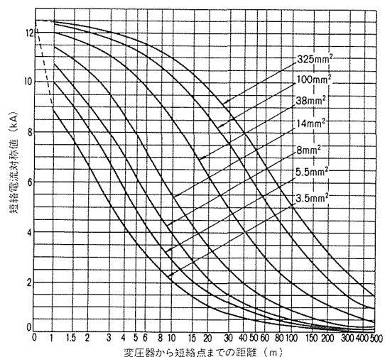
付図6 三相変圧器容量100kVA、二次電圧200V
