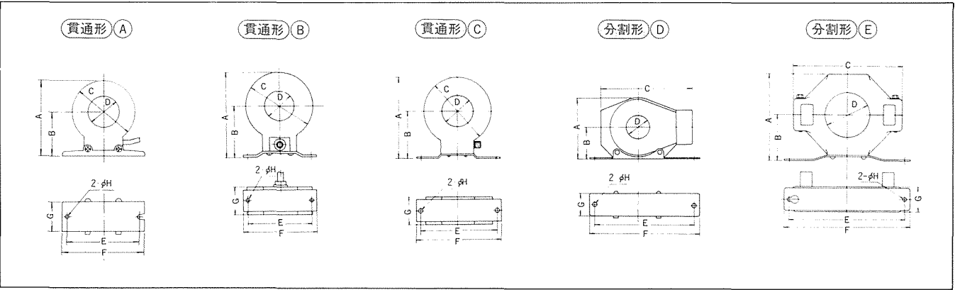
■変流器外形寸法表
