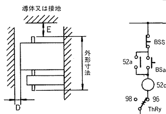
標準接続図
