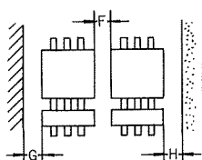
取付間隔
