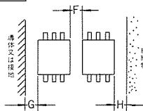
取付間隔
