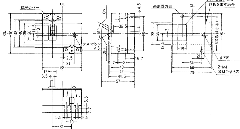
穴明寸法
