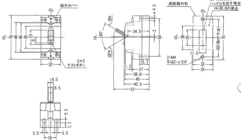
穴明寸法
