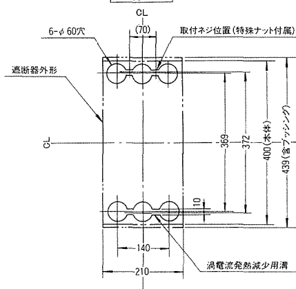
穴明寸法
