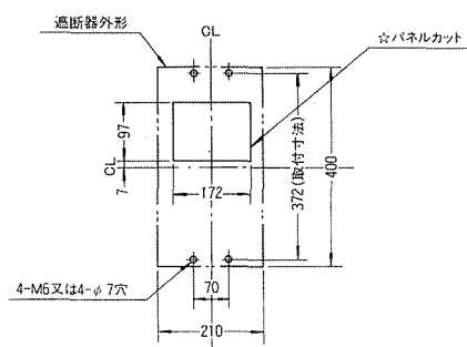
穴明寸法
