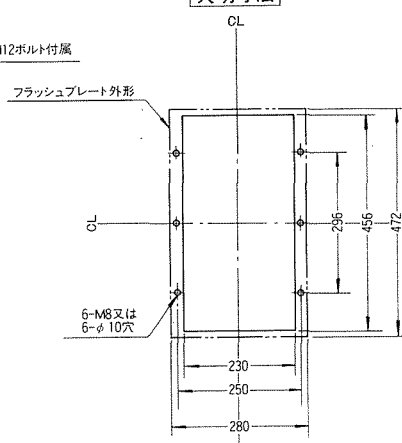
穴明寸法
