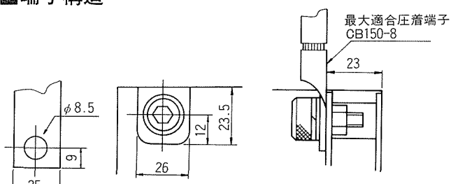
導帯加工図 (最大)
