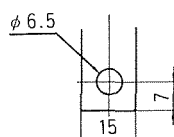
導帯加工図 (最大)
