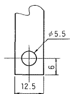
導帯加工図 (最大)
