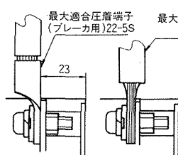
導帯・圧着端子接続
