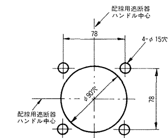
扉穴明加工図
