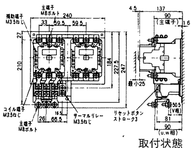
取付状態
