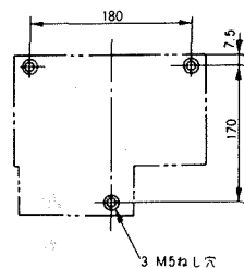
穴明寸法
