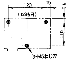
穴明寸法
