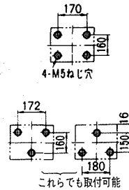
穴明寸法
