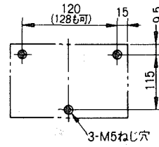
穴明寸法
