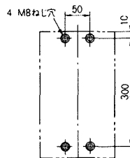
穴明寸法
