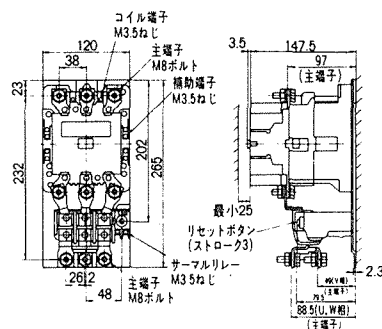
取付状態
