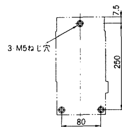
穴明寸法
