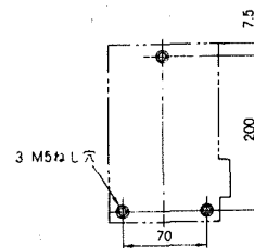
穴明寸法
