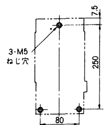
穴明寸法
