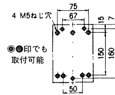
穴明寸法
