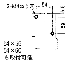
穴明寸法
