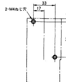
穴明寸法
