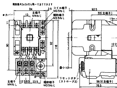
取付状態
