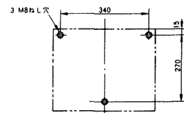
穴明寸法
