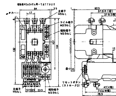
取付状態
