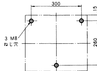
穴明寸法
