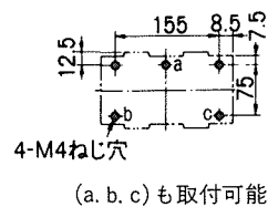
穴明寸法
