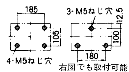
穴明寸法
