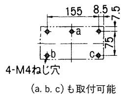
穴明寸法
