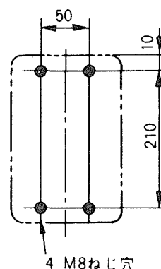
穴明寸法
