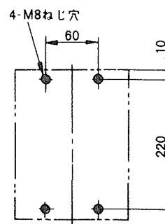
穴明寸法
