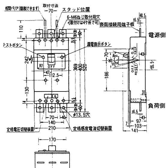
埋込形
