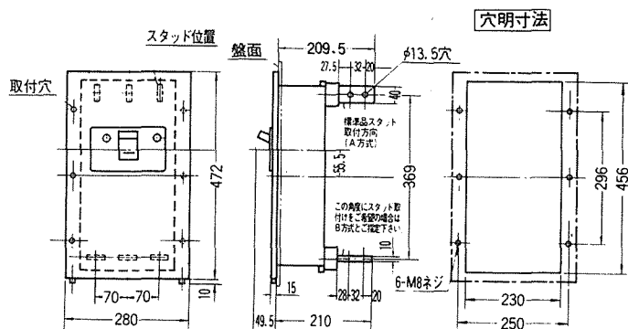
埋込形
