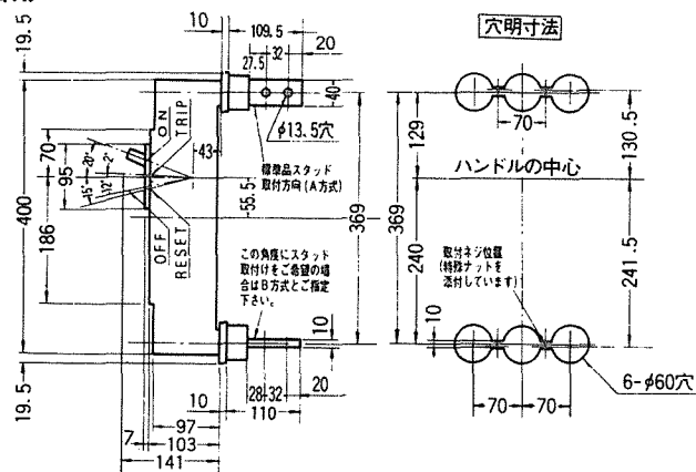
埋込形
