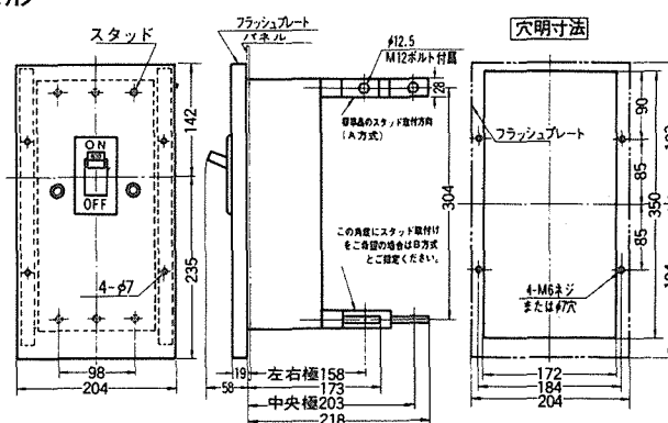
埋込形
