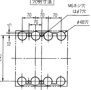
穴明寸法
