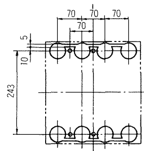
穴明寸法
