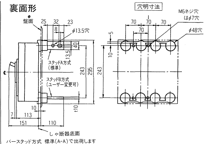
穴明寸法
