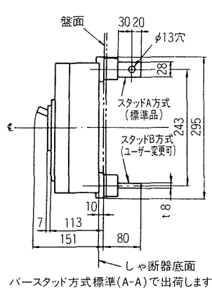
裏面形
