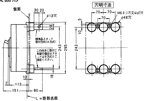
裏面形
