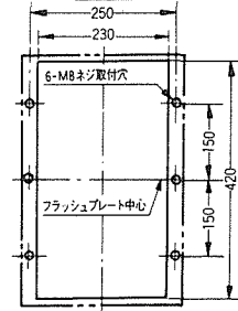
穴明寸法
