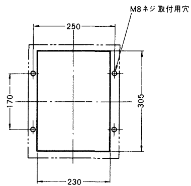
穴明寸法
