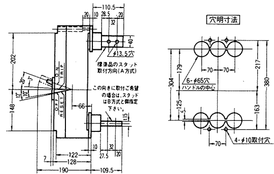
裏面形
