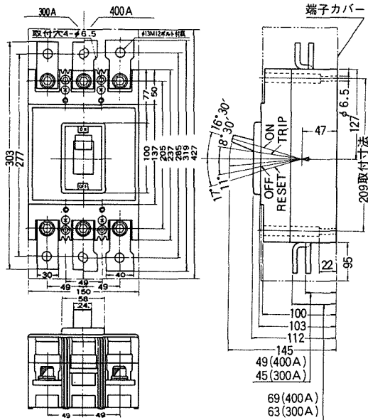
埋込形
