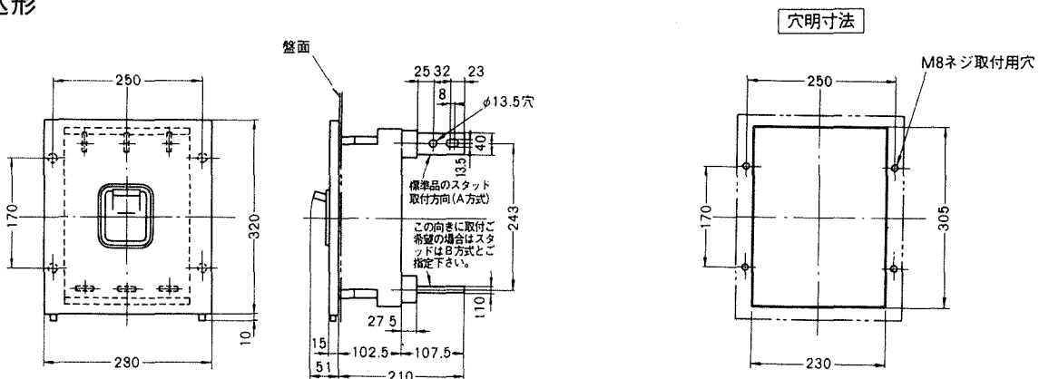
埋込形
