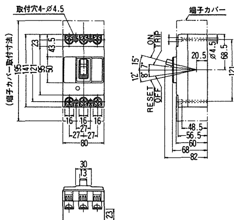
埋込形
