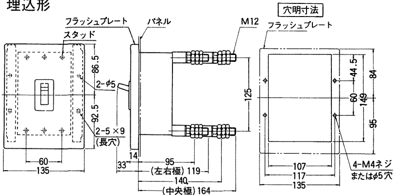
埋込形
