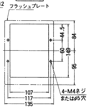
穴明寸法
