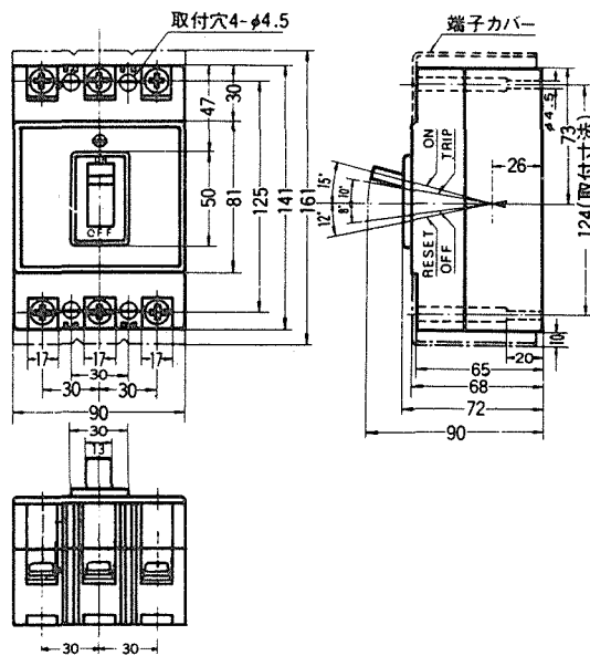
埋込形
