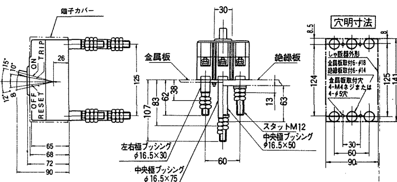
裏面形
