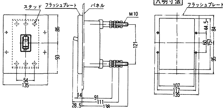
穴明寸法
