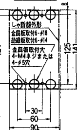
穴明寸法
