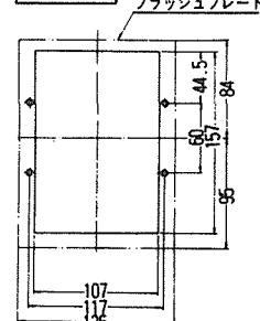
穴明寸法
