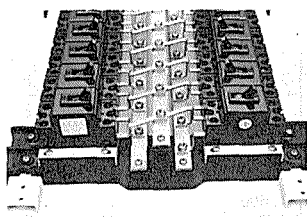
100V配線
