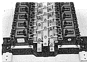
200V配線
