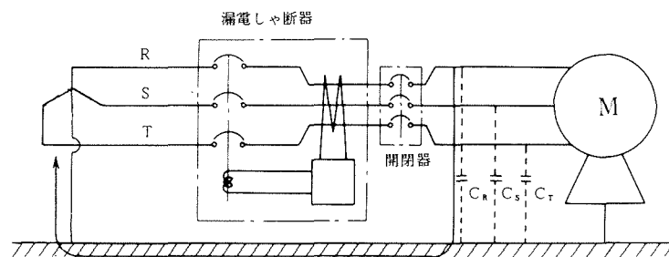
不揃い投入しゃ断による誤動作
